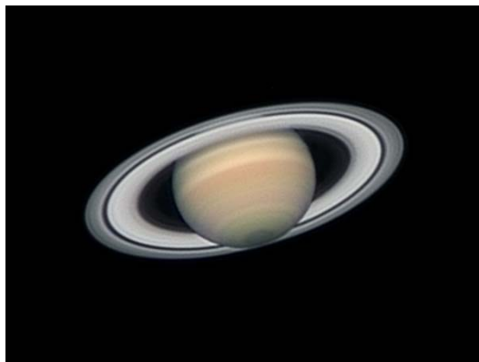
土星イメージ
