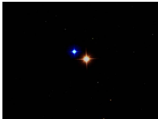
白鳥座「アルビレオ」イメージ
