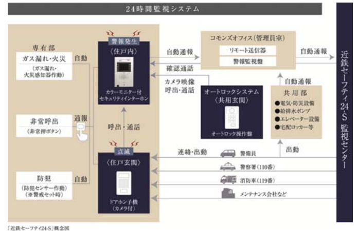
【セキュリティシステム概念図(近鉄セーフティ24S)】
