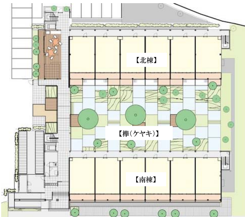
【敷地配置図】
