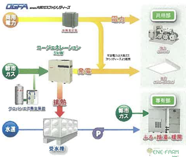
防災対応型マンションコージェネシステム概念図
